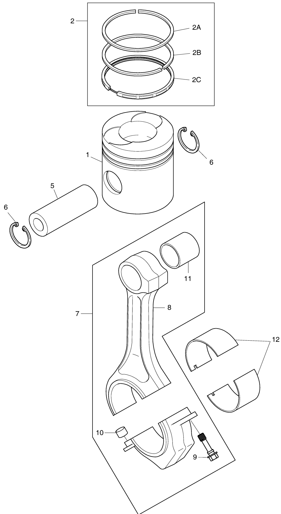
Fig. 016 PISTON ASS'Y
