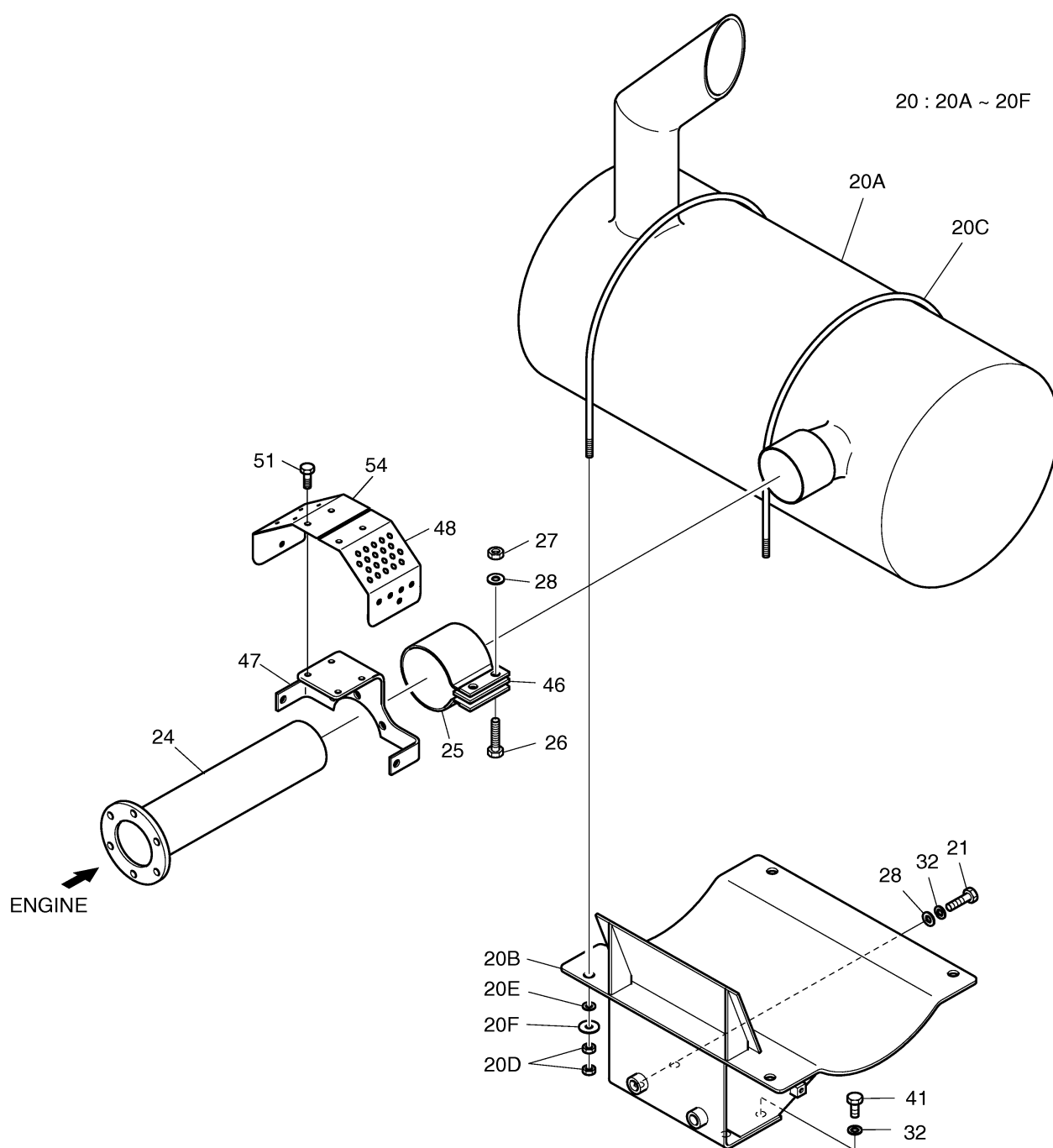
Fig. 1150 MUFLER
