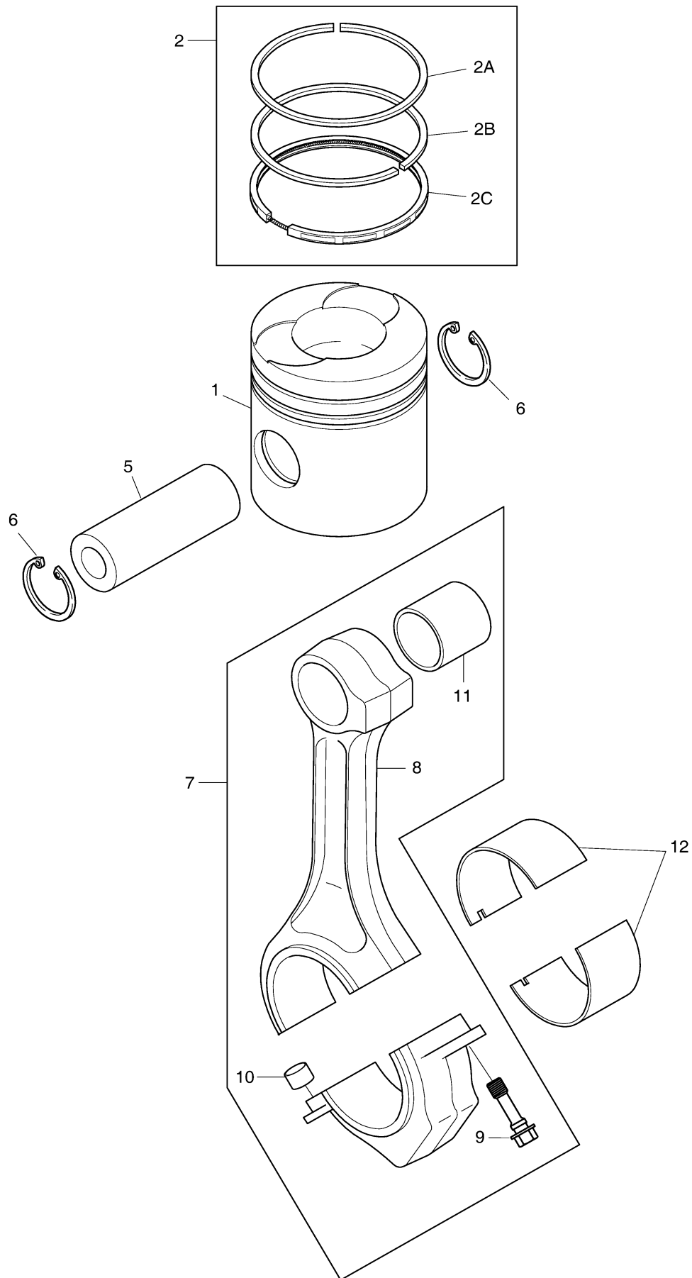
Fig. 016 PISTON ASS'Y
