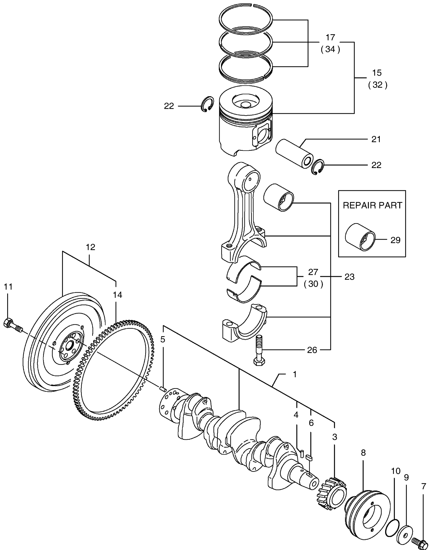
Fig. 018 CRANK SHAFT & PISTON
