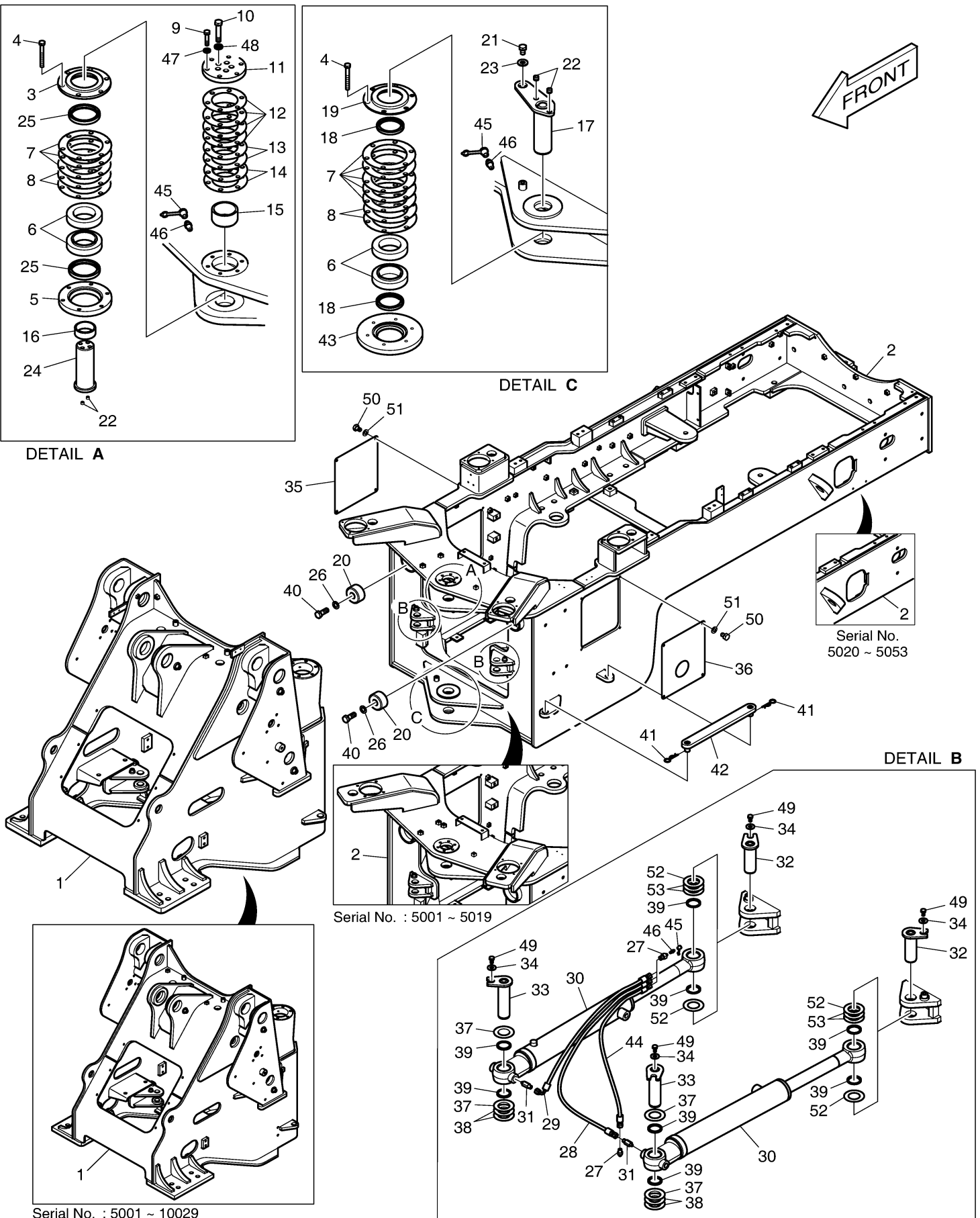
Fig. 1100 FRAME
