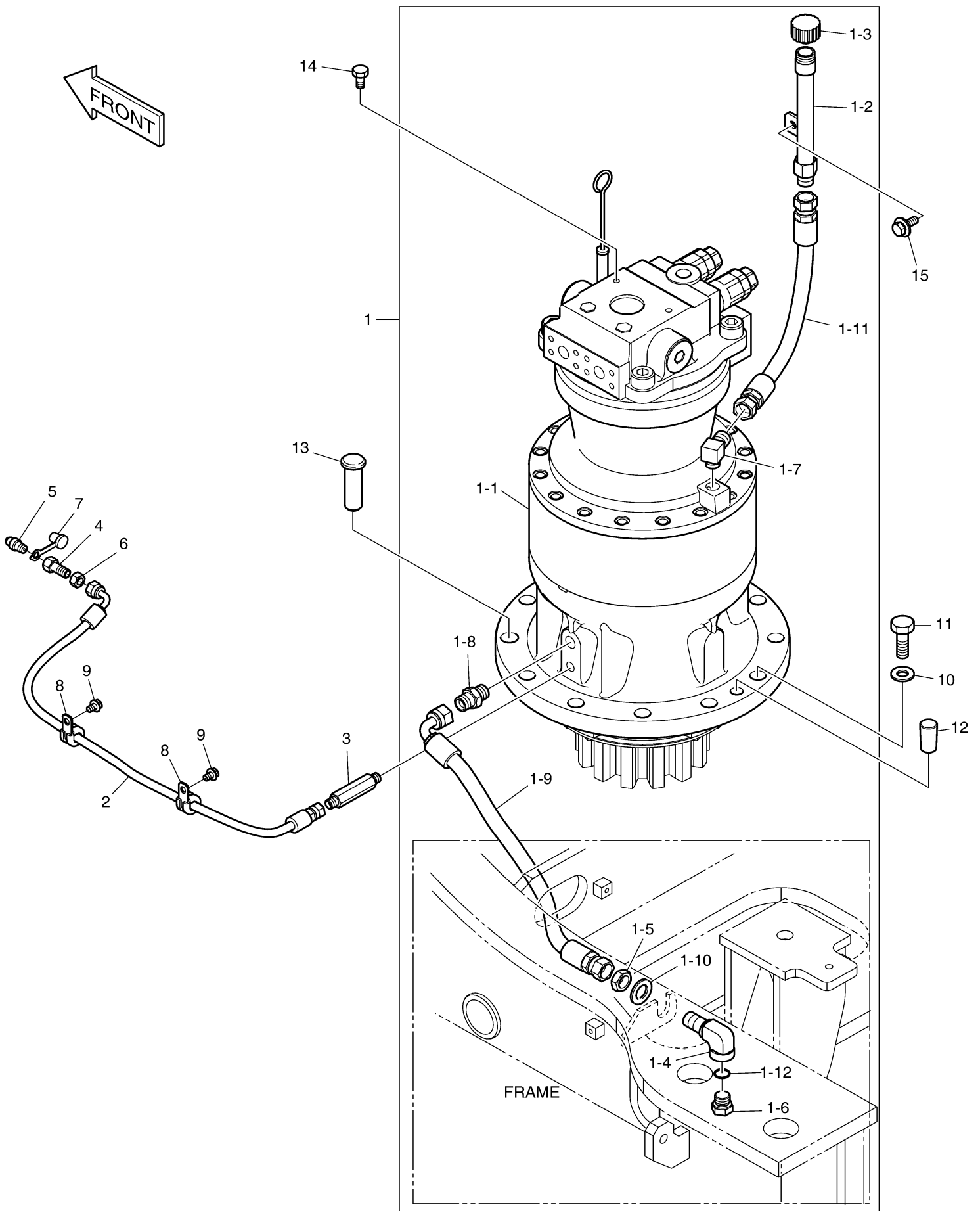
Fig. 1190 SWING MOTOR
